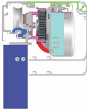
şık GEZE Design formunda yuvarlatılmış kapak profili
